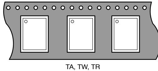
Figure 44. WLCSP 3-, 4-, 6-, 8-, 10-, & 12-Bump
